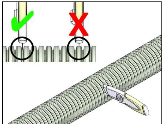
Abb. 3: Flexrohr ablängen
